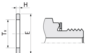
торцевое уплотнение для штуцеров типа COM-G
